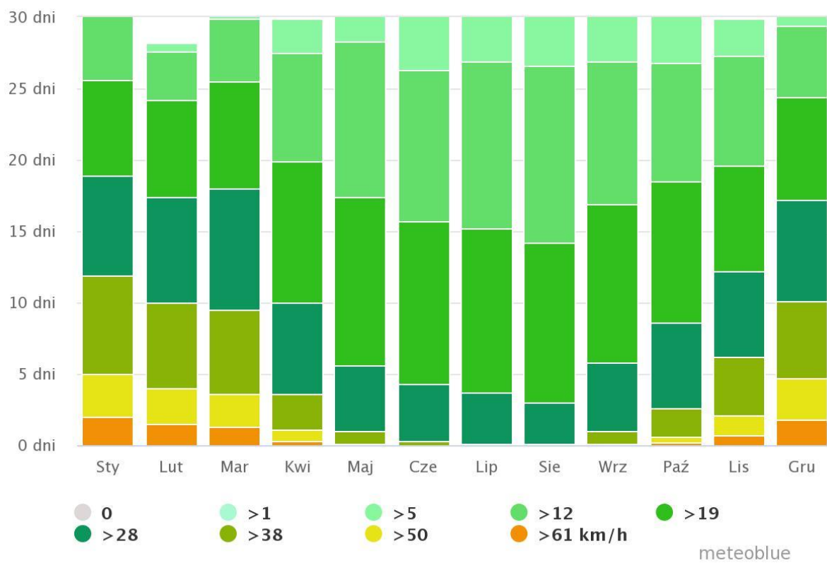
Rycina 6. Wykres prędkości wiatru dla Miasta Sławków
