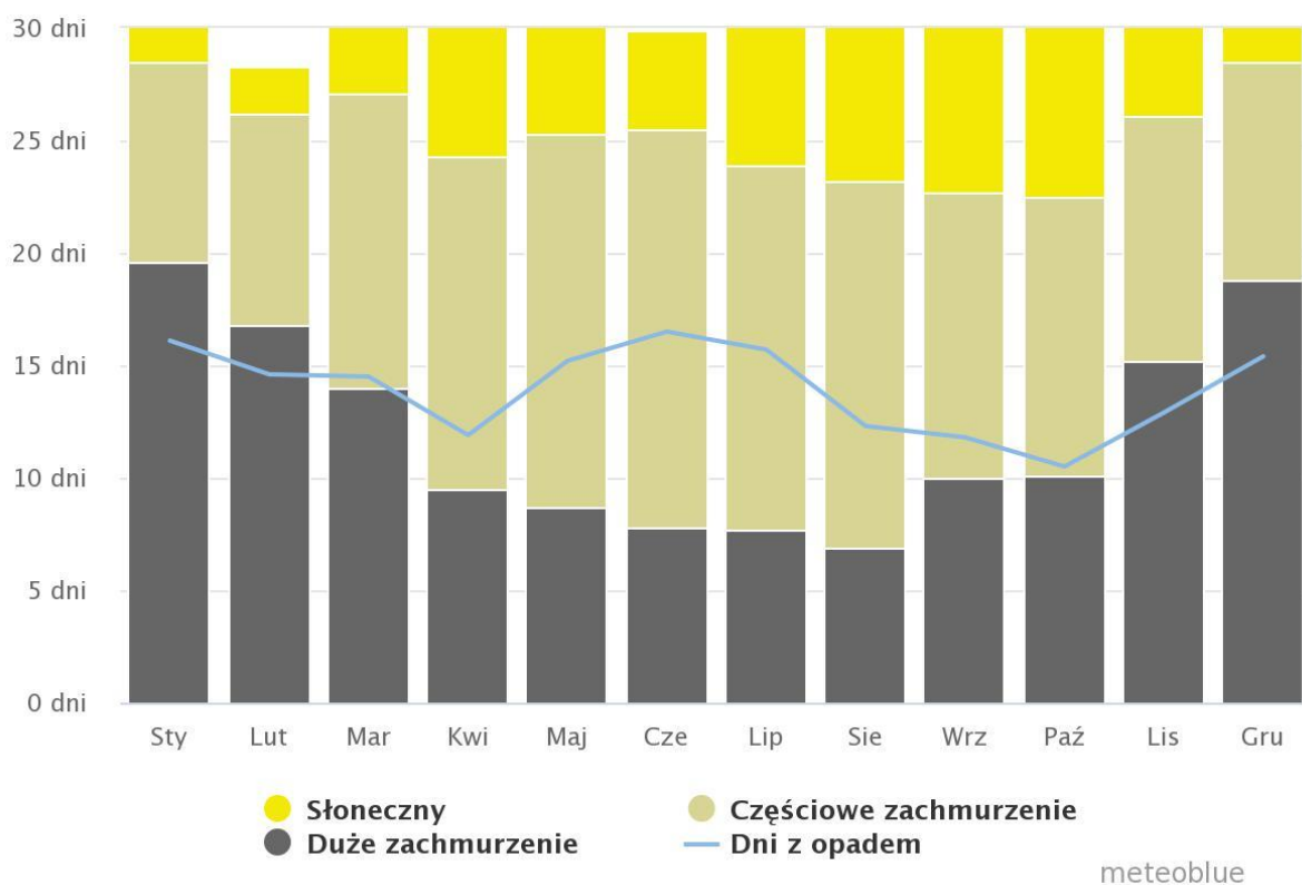
Rycina 4. Wykres dni o dużym zachmurzeniu, słonecznych i z opadami dla Miasta Sławków
