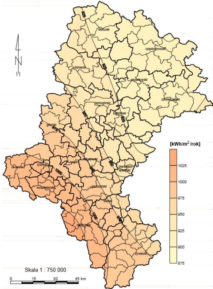
RYSUNEK 11. POTENCJAŁ ENERGETYKI SŁONECZNEJ NA TERENIE WOJEWÓDZTWA ŚLĄSKIEGO. Źródło: Projekt Programu wykorzystania odnawialnych źródeł energii na terenach nieprzemysłowych województwa śląskiego.
